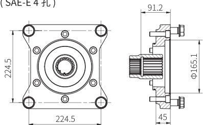
型号 C241L (SAE-E 4 孔)
