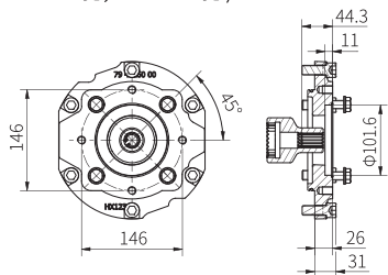
型号 C238L (SAE-C 2 孔; SAE-C 4 孔)
