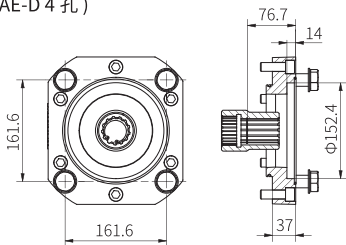
型号 C249L (准备用于串联泵的通轴（盖）)
