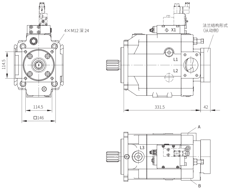
外壳结构形式 -2（纵向接口，带通轴）
