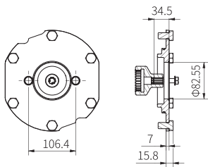
型号 C235L (SAE-B 4 孔)
