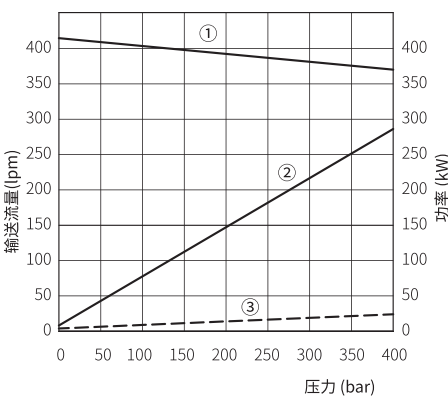
型号 V30E - 270, V30EL - 280
